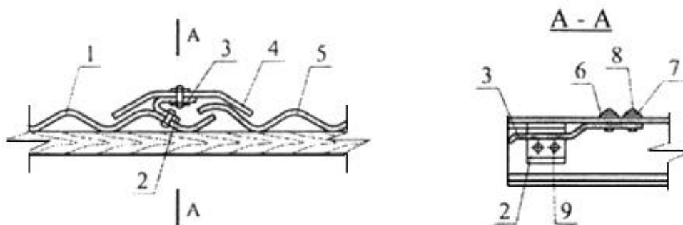
Рисунок Н.3 - Компенсационный шов
