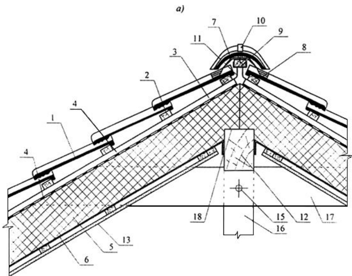
Рисунок И.2 - Конек крыши с одним вентиляционным зазором и конек кровли с чердаком и вентиляционным элементом в гидрозащитной пленке
