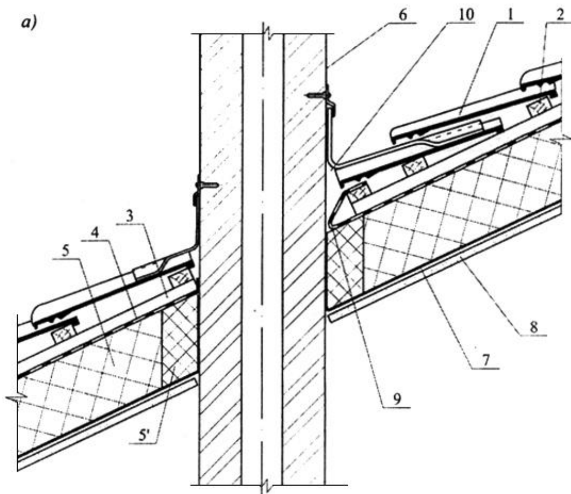
Рисунок И.4 - Сопряжение крыши с трубой и стеной
