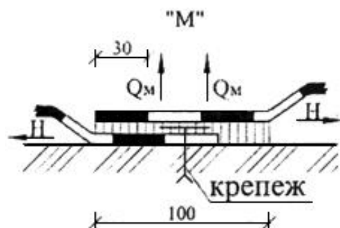
Рисунок Е.5 - Силы, действующие в точке М
