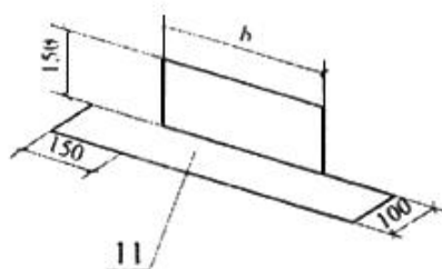
Передний уголок (b - ширина трубы)
