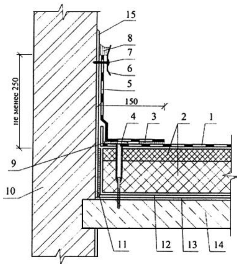
Рисунок Ж.9 - Примыкание кровли к стене
