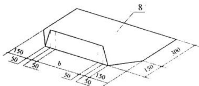
Уголок со стороны конька (b - ширина трубы)
