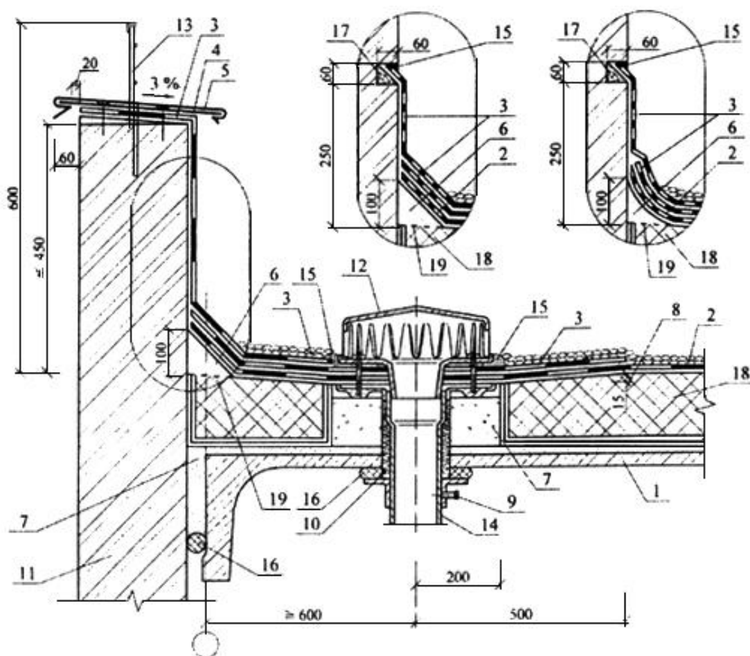
Рисунок Ж 1 - Воронка у примыкания кровли к парапету
