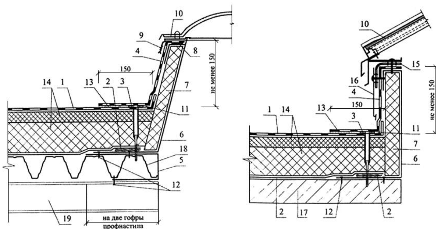
Рисунок Ж.6 - Примыкание кровли к зенитному фонарю
