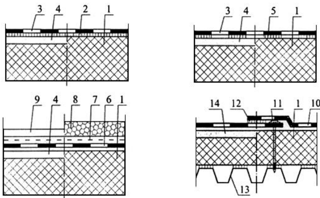
Рисунок Е.1 - Способы укладки кровельного ковра
