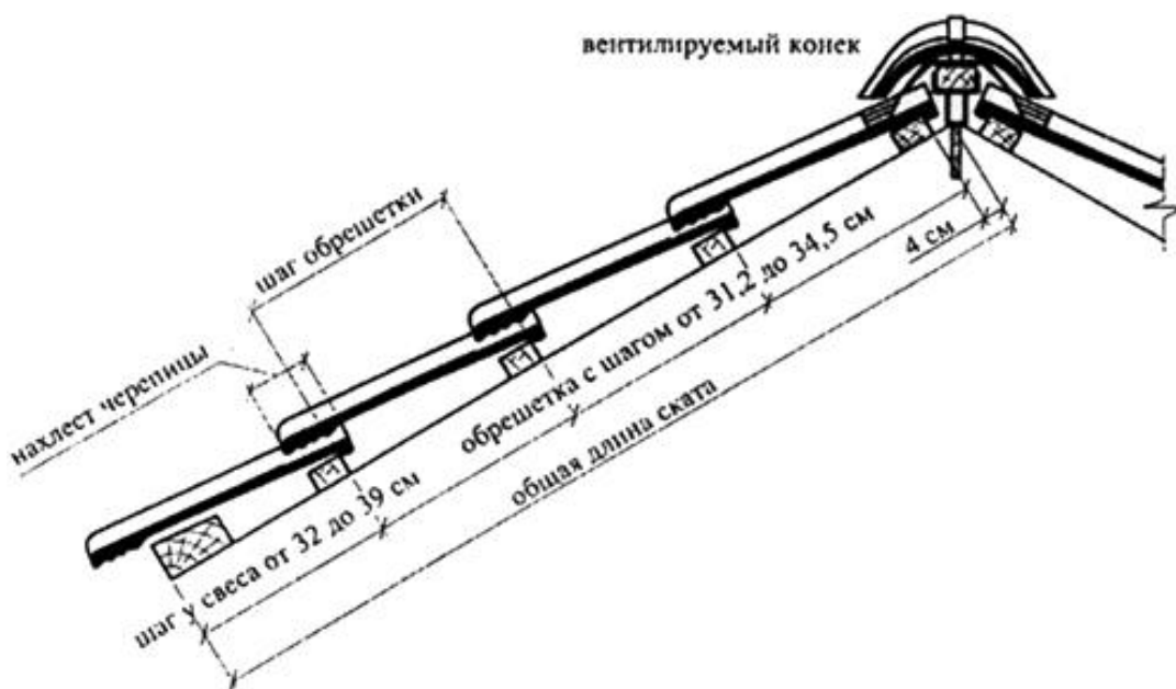
Рисунок К.1 - Поперечный разрез черепичной кровли
