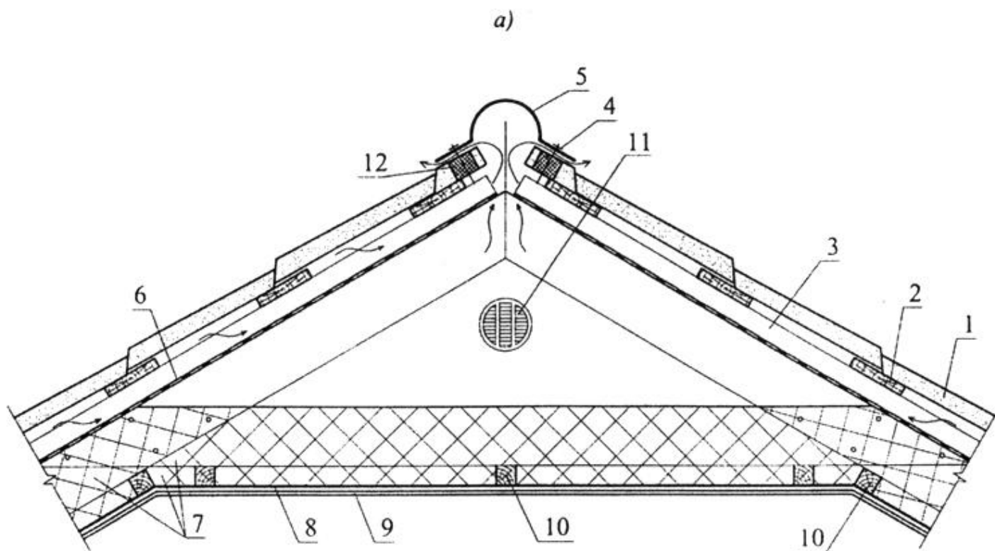
Рисунок П.2 - Коньковый узел кровли с вентиляцией через коньковый элемент и через вытяжную трубу
