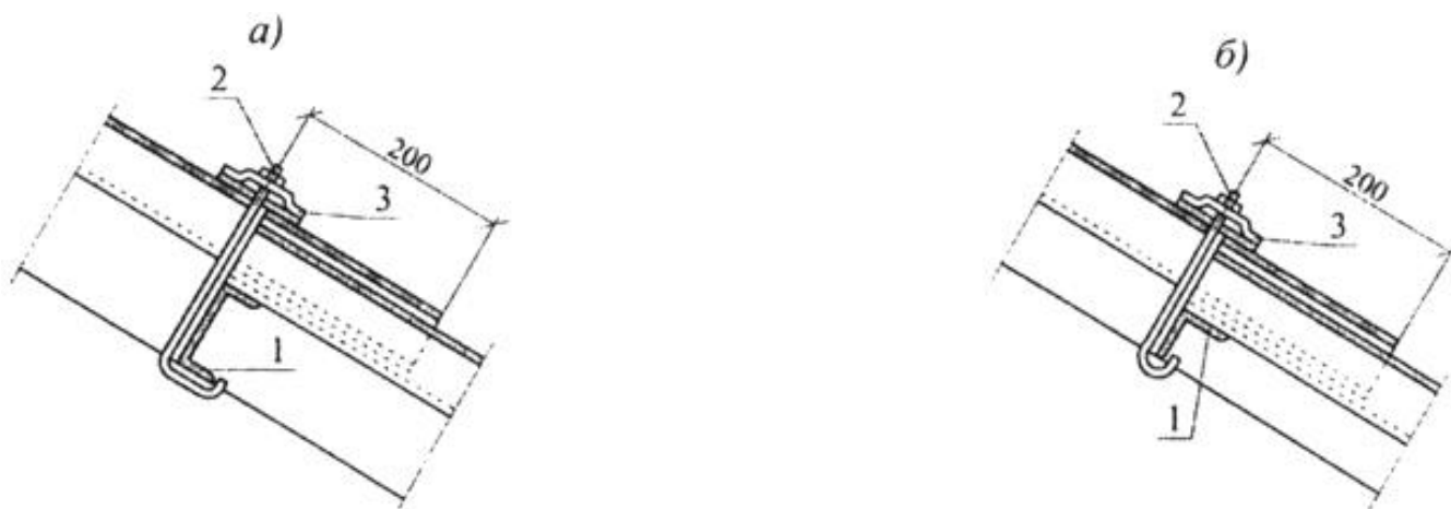
Рисунок Н.4 - Крепление волнистых листов к металлическим прогонам из швеллера и уголка
