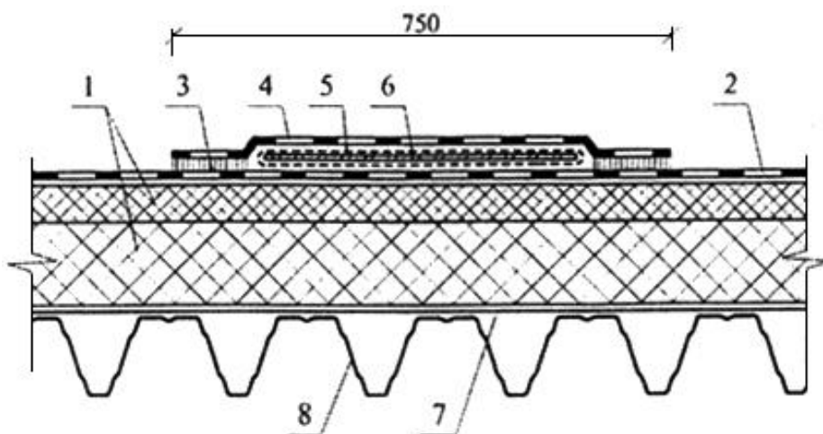
Рисунок Ж.8 - Ходовая дорожка
